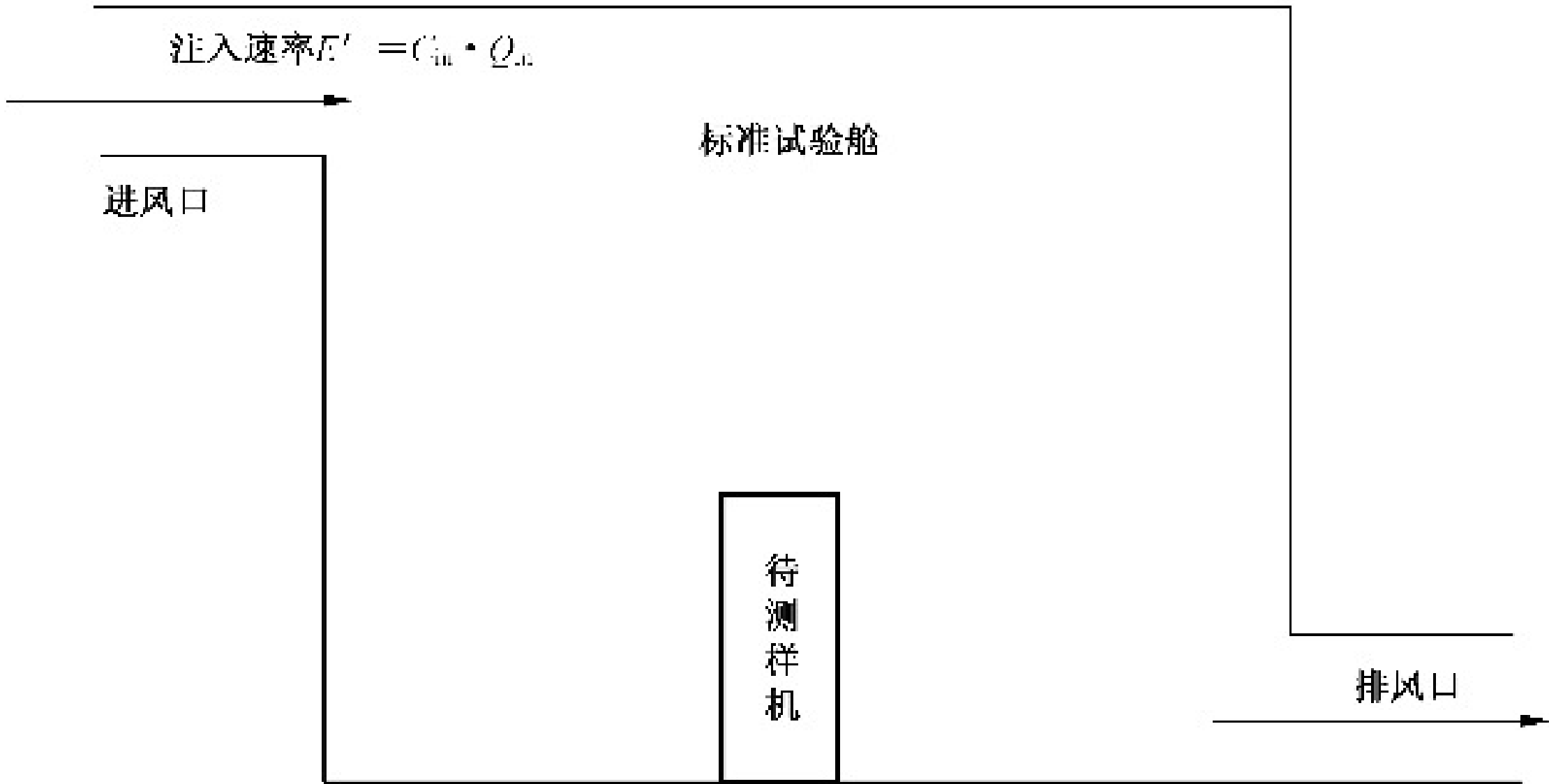
图 O.1 臭氧测试示意图
