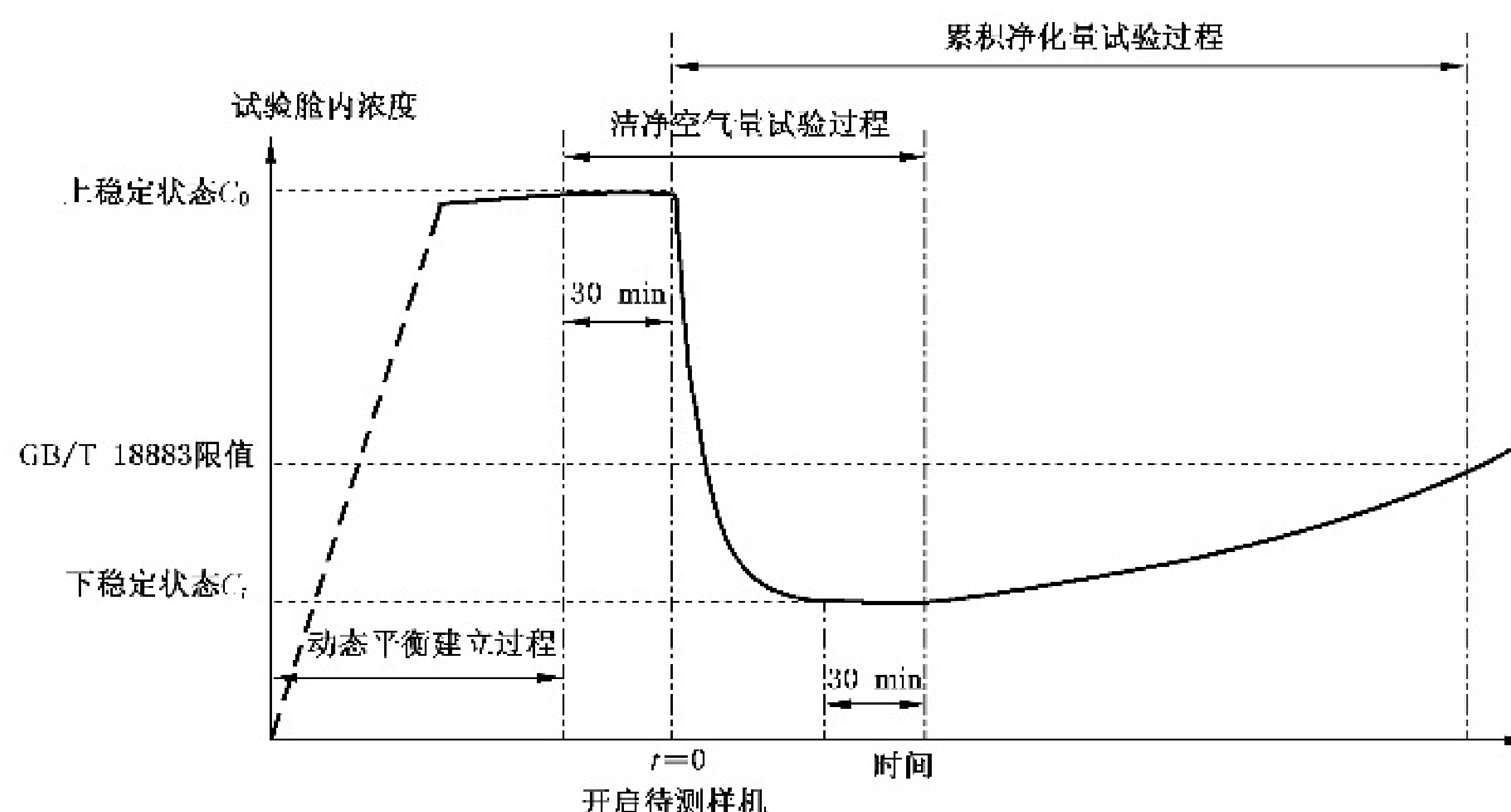
图 0.2 动态平衡试验原理图
