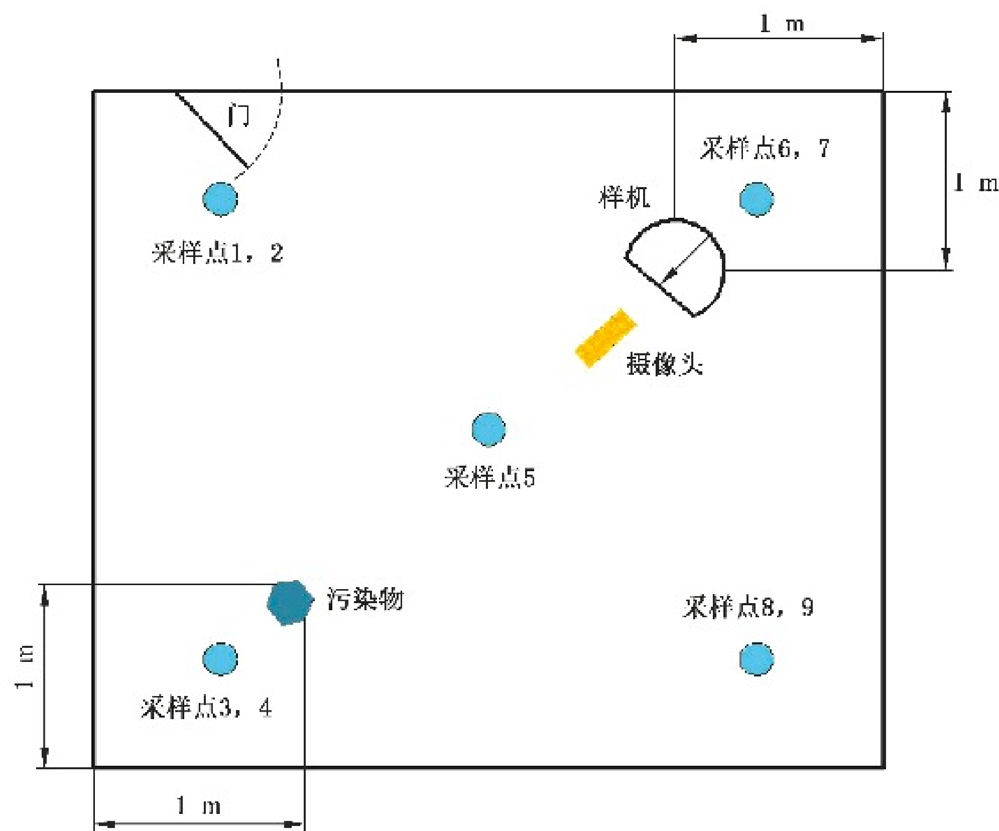
图 K.1 试验舱布局示意图
