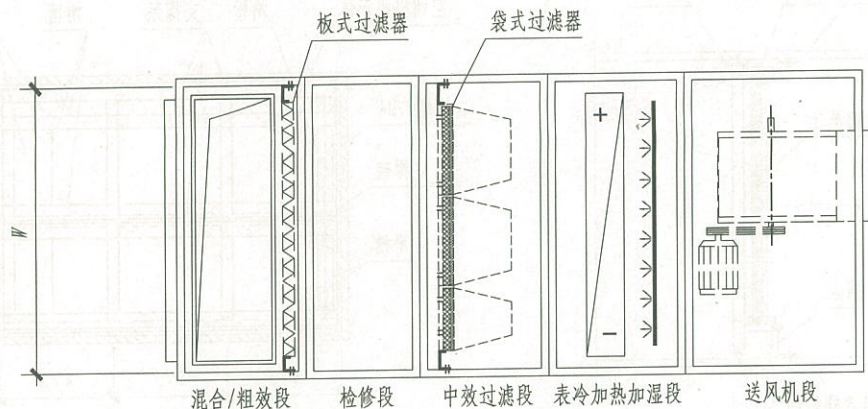
平面图
