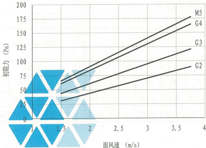
板式加强筋式过滤器初阻力—面风速曲线图
