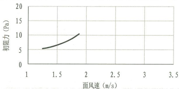
EP01-FC-07过滤器初阻力—面风速曲线图
