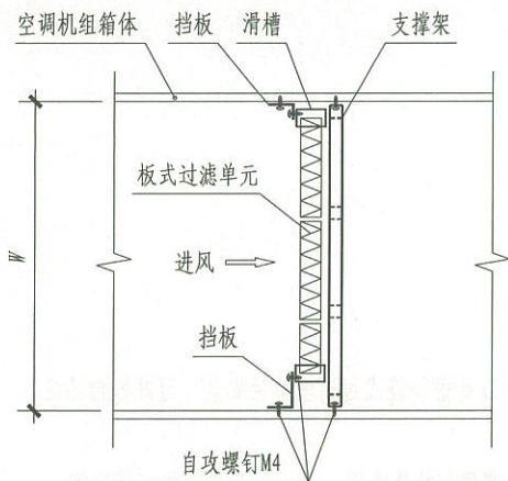
板式过滤单元安装平面图
