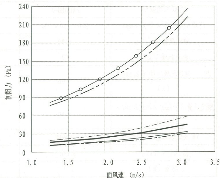
EP-AC-02过滤器初阻力一面风速曲线图
