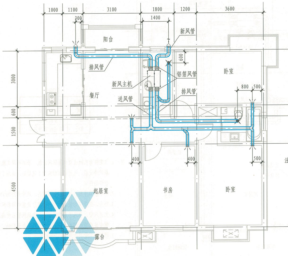
住宅集中新风机布置案例一
