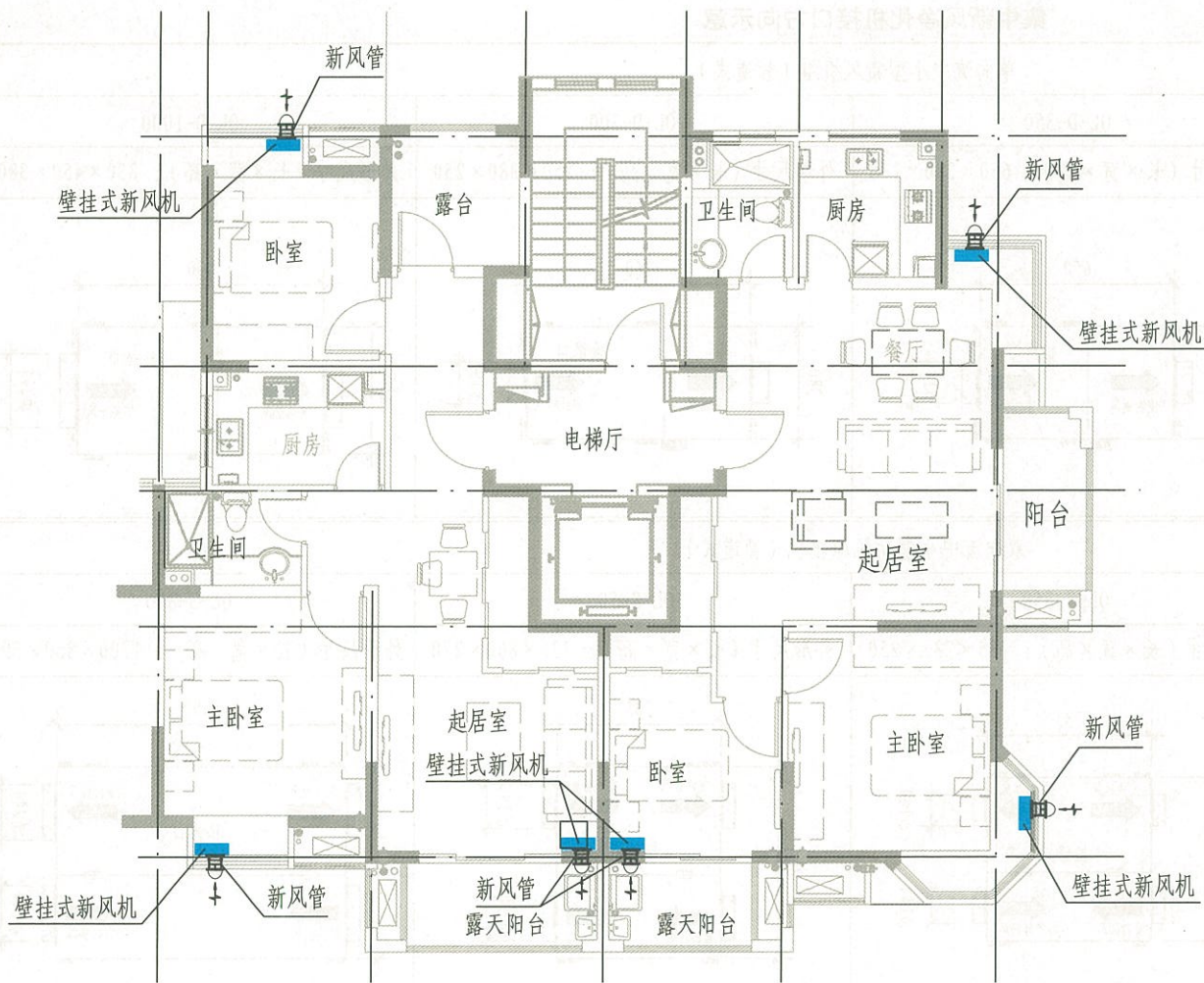
住宅独立新风净化机布置案例
