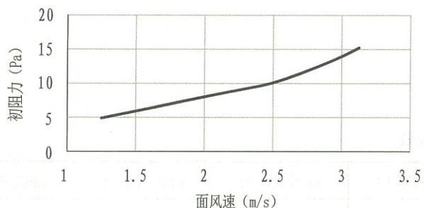
EP01-FC-01过滤器初阻力—面风速曲线图
