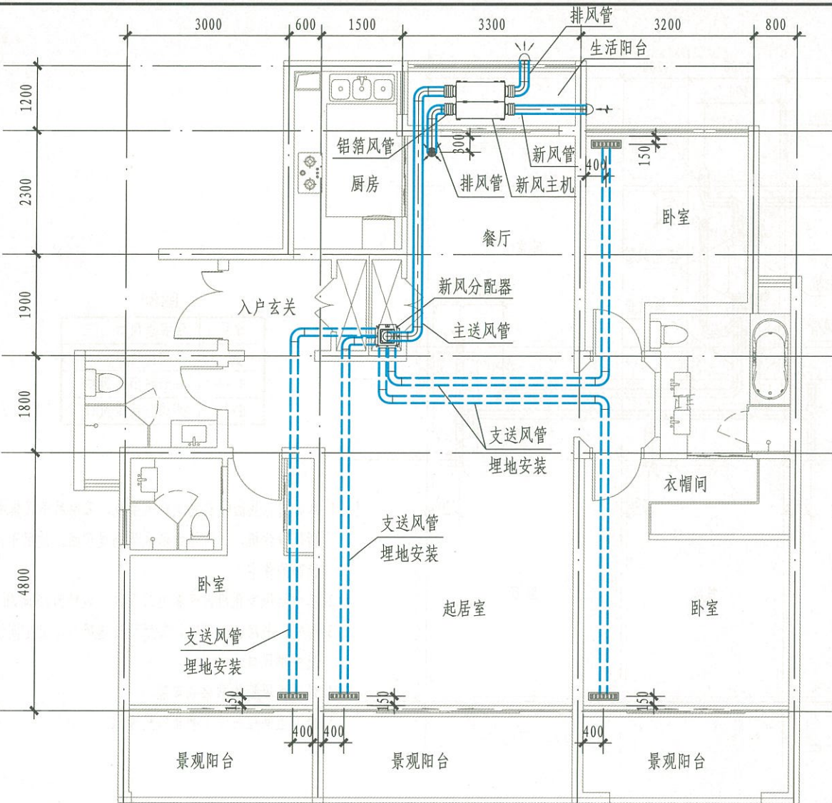
住宅集中新风净化机布置案例
