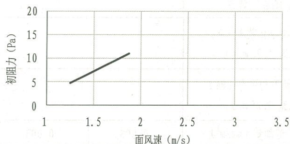
EP01-FC-06过滤器初阻力—面风速曲线图
