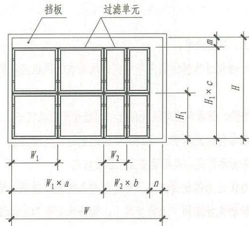
过滤单元机组内布置示意图
