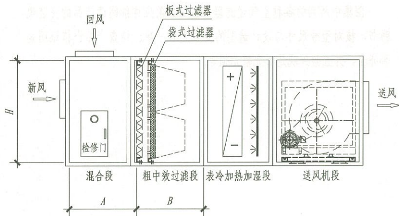
立面图
