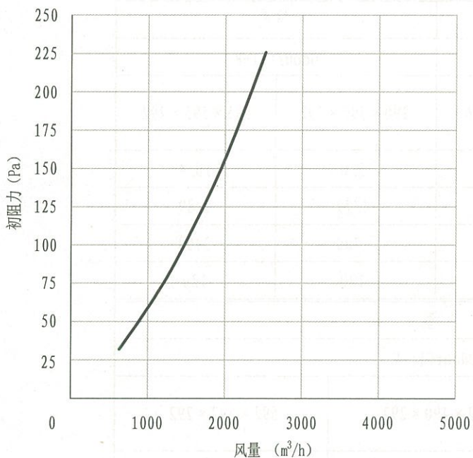
Odourfil-D型活性炭过滤器初阻力—风量曲线图
