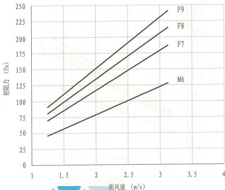
板式无隔板过滤器初阻力—面风速曲线图
