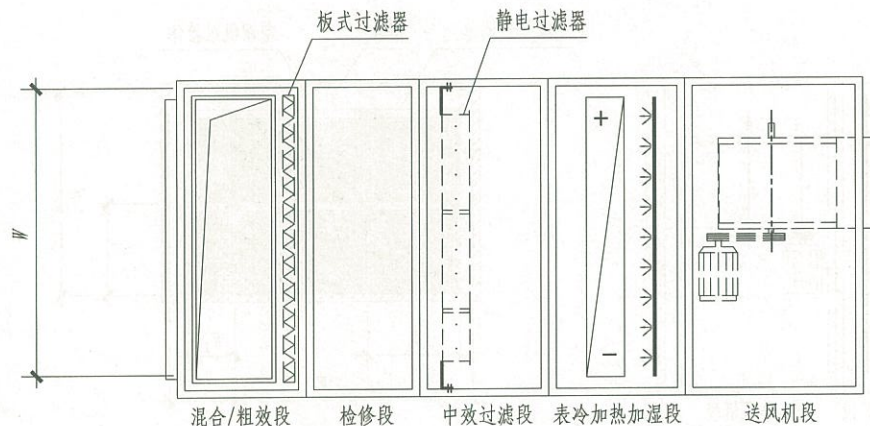
平面图
