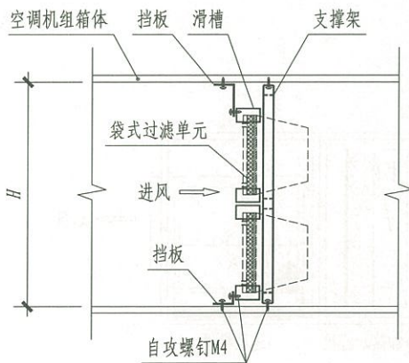
袋式过滤单元安装立面图
