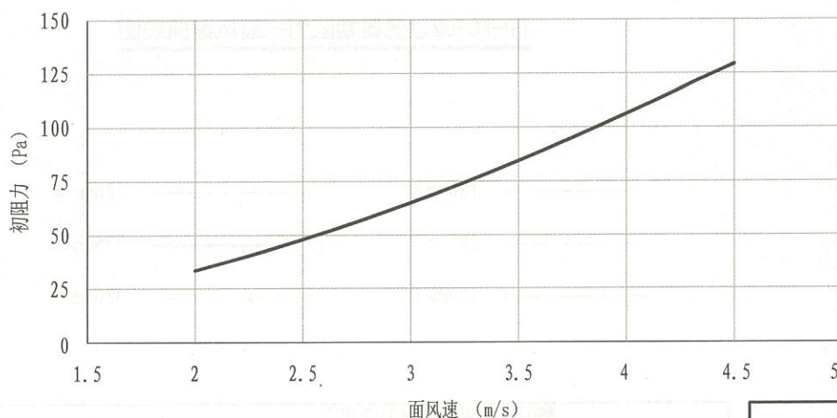
FAH01M-A过滤器初阻力—面风速曲线图
