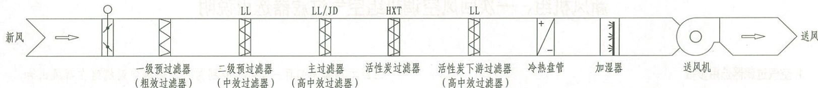
新风机组空气过滤器设置流程图
