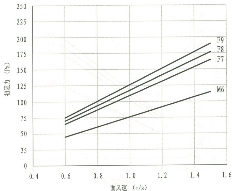
150mm厚板式有隔板过滤器初阻力—面风速曲线图
