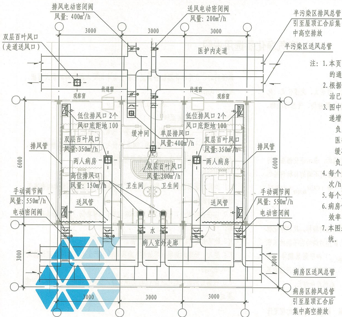
应急医院两人间负压病房通风系统设计平面示意图
