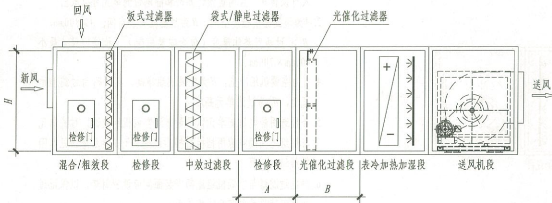
立面图
