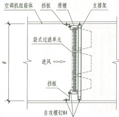
袋式过滤单元安装平面图
