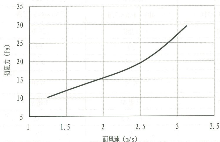
EP-DS-01过滤器初阻力—面风速曲线图
