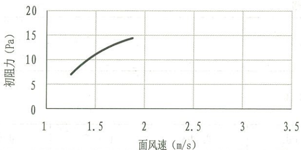
EP01-FC-05过滤器初阻力—面风速曲线图
