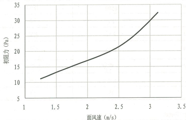
EP-DS-02过滤器初阻力—面风速曲线图
