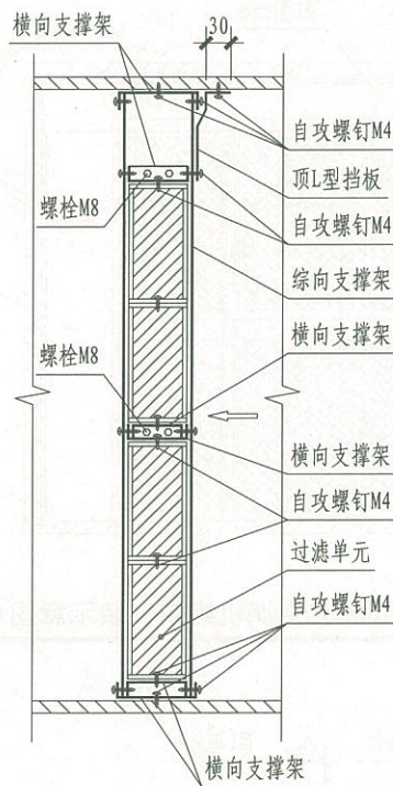
A-A剖面图
