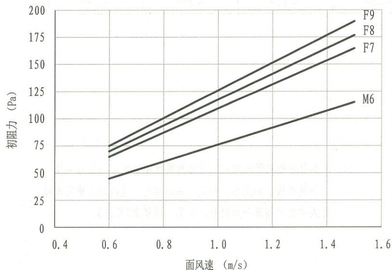
V型板式过滤器初阻力一面风速曲线图
