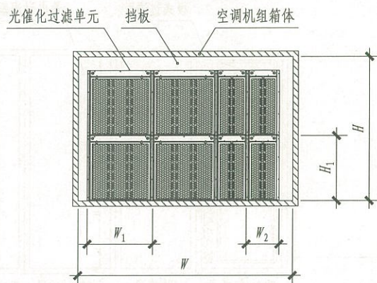
光催化过滤单元机组内布置示意图
