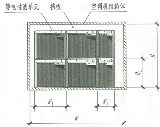
静电过滤单元机组内布置示意图
