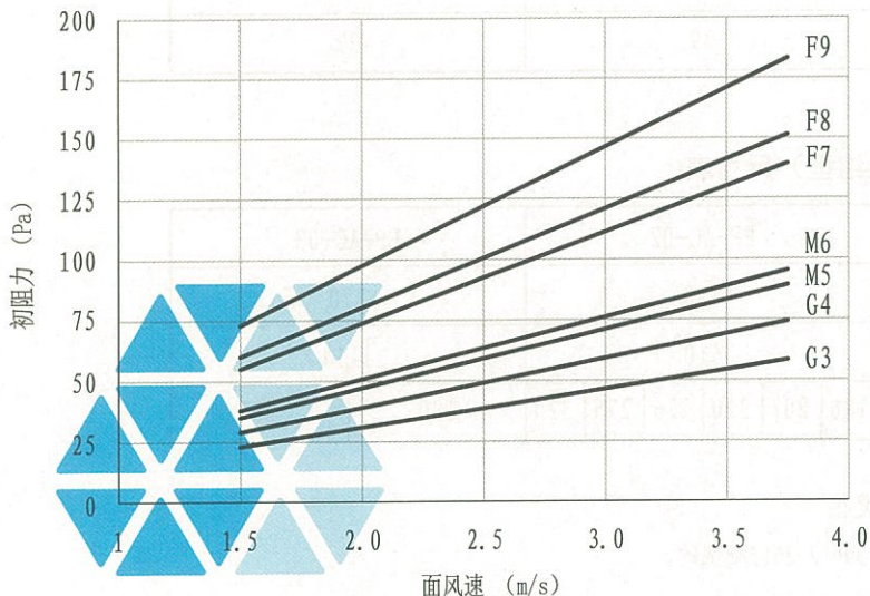
袋式过滤器初阻力—面风速曲线图
