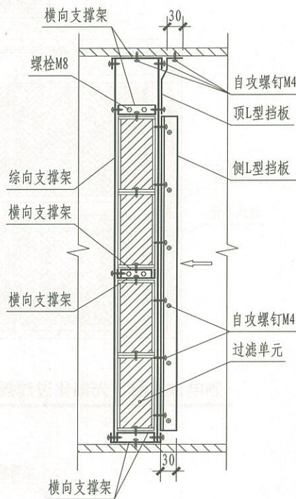
B-B剖面图
