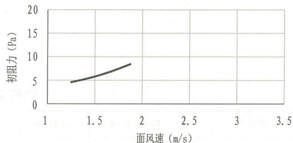
EP01-FC-04过滤器初阻力—面风速曲线图
