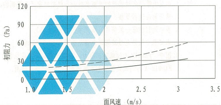
EP-AC-03过滤器初阻力一面风速曲线图
