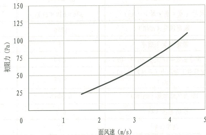
FAD01M-A过滤器初阻力—面风速曲线图
