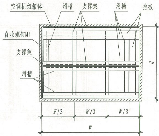
板式、袋式过滤器安装框架示意图
