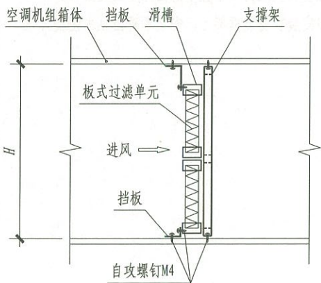
板式过滤单元安装立面图
