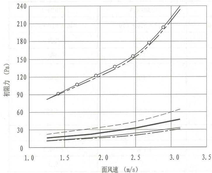
EP-AC-01过滤器初阻力一面风速曲线图
