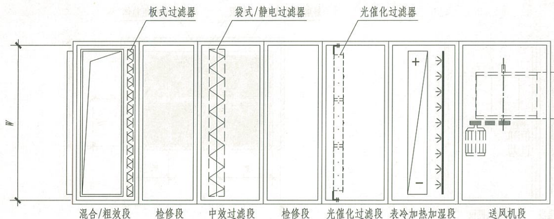
平面图
