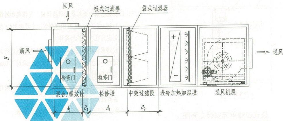
立面图
