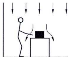
图 A.3 人员和物体对单向流的影响
